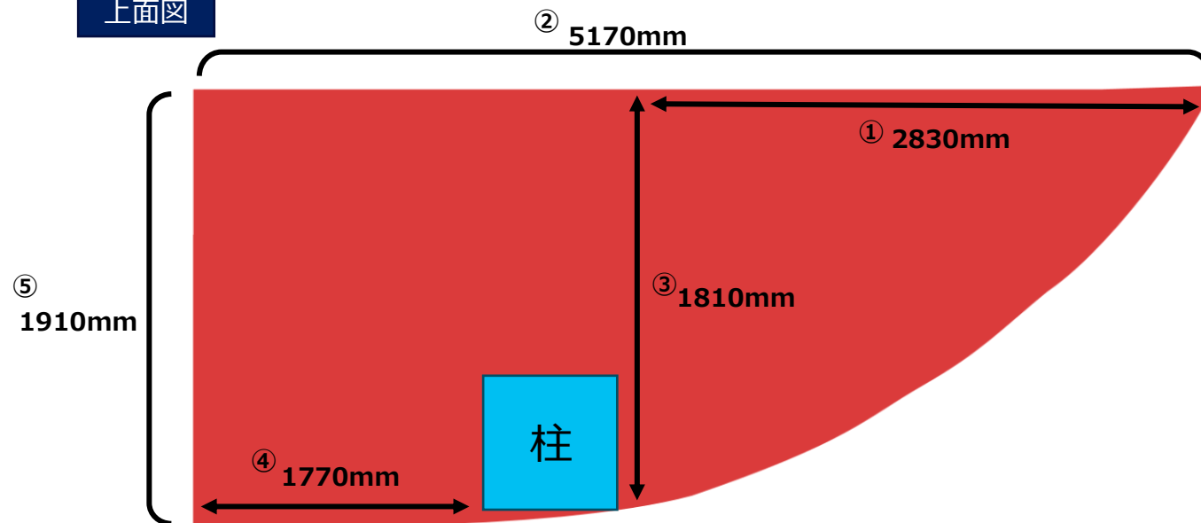
上面図
